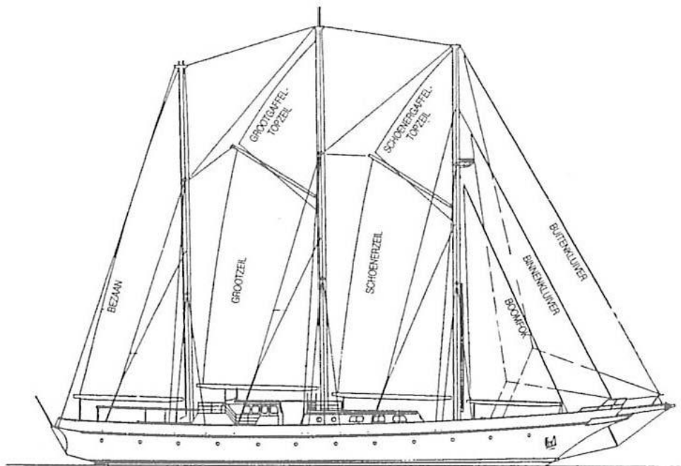
Het zeilplan
